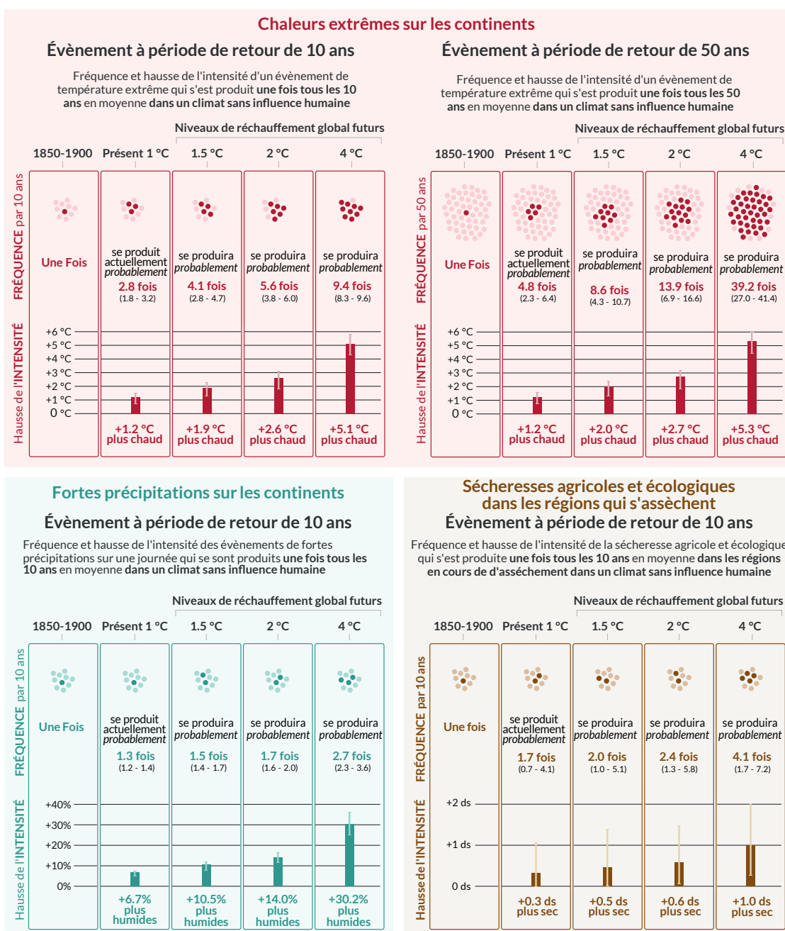
Figure 9 : Evolution des extrêmes de température, précipitation et sécheresses. La figure montre le changement de fréquence ou le changement d'intensité, pour un climat plus chaud, en partant d'un évènement qui se produisait une fois tous les 10 ou 50 ans dans le climat de la période préindustrielle. Dans la partie supérieure, chaque point représente une année. Les points de couleur sombre indiquent les années où un évènement d'intensité égale ou supérieure à celle de la période pré-industrielle se produit (augmentation de fréquence à seuil d'intensité constant). Pour plus d'information, voir la légende de la figure source : SPM.6.
