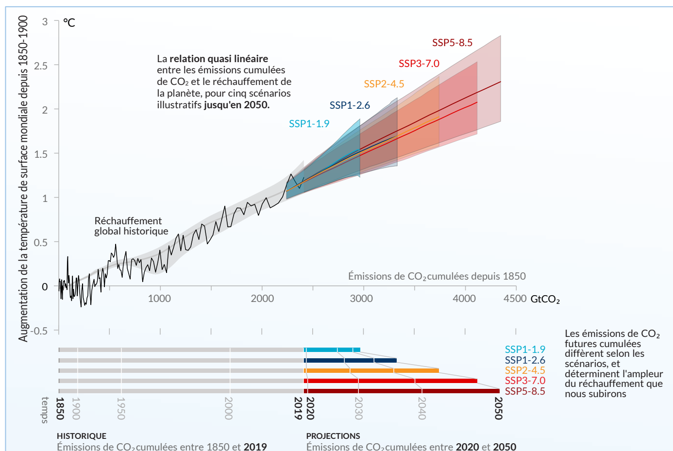
Figure 7 : Les données historiques (ligne noire fine) montrent l'augmentation observée de la température moyenne en surface depuis 1850-1900 en fonction des émissions historiques cumulées de dioxyde de carbone, de 1850 à 2019. Les zones colorées indiquent la fourchette de projections de la température moyenne en surface jugée très probable, et les lignes centrales colorées indiquent l'estimation médiane en fonction des émissions cumulées de CO 2 , de 2020 à 2050 pour l'ensemble des scénarios illustratifs (voir question 6). Les données s'arrêtent en 2050 parce que au-delà de cette date, les émissions sont négatives (absorption nette) pour certains scénarios, or il y a peu de preuves que la proportionnalité illustrée ici persiste dans cette situation. Traduction réduite et adaptée ; pour la légende complète, voir la source : figure SPM.10.
