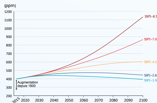
Figure 5c : Concentration en CO 2 dans l'atmosphère (d'après Meinshausen, M. et al. 2020: doi.org/10/gg8vs4)
