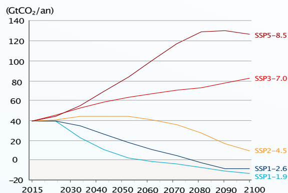
Figure 5b : Émissions de CO 2 (figure SPM4.a)
