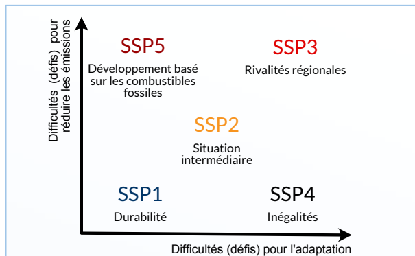
Figure 5a: Trajectoires communes d'évolution socio-économique [33]
