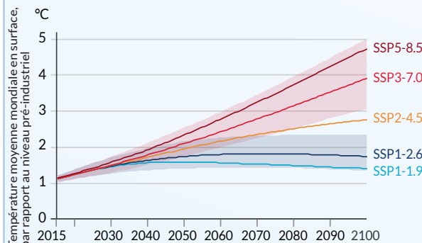
Figure 5d: Température moyenne mondiale en surface pour un ensemble des modèles. Les plages de couleurs claires indiquent la gamme «très probable» (probabilité > 90%) pour SSP3-7.0 et SSP1-2.6 (fig. SPM.8)
