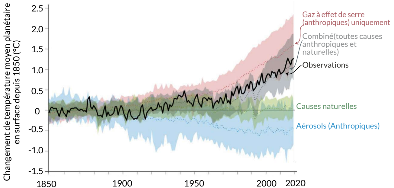
Figure 2. Le réchauffement observé (1850-2018) n'est reproduit que dans les simulations qui incluent l'influence humaine.
